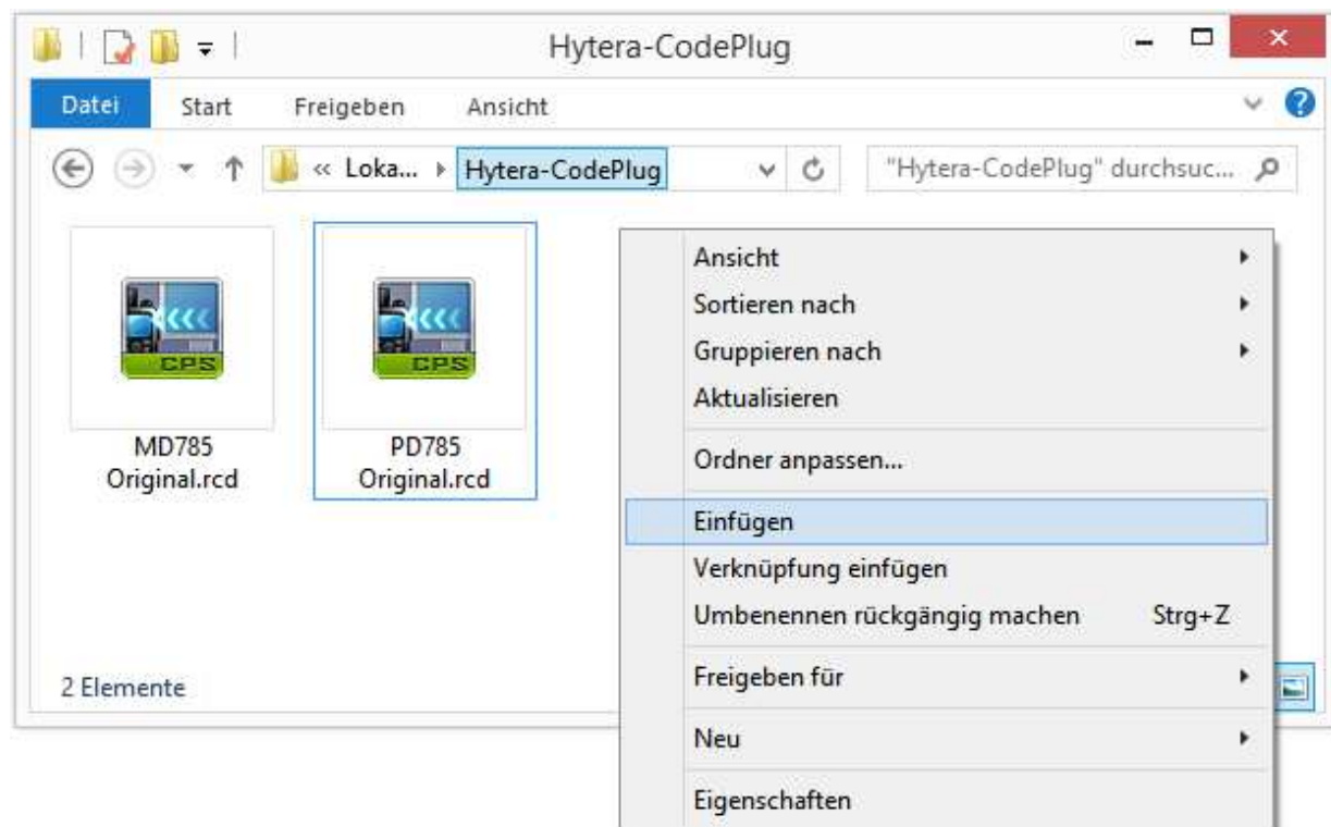
Rys. C.3. Wklejenie pliku
