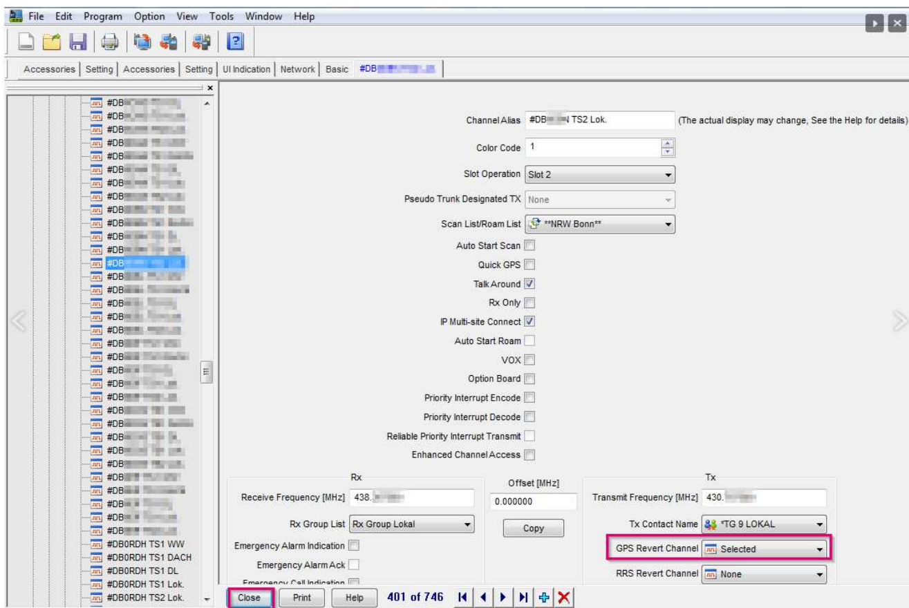
Rys. 5.31. Konfiguracja GPS – pole „GPS revert channel” dla wybranego kanału w szczelinie 2. Dla kanałów pracujących w szczelinie 1 wybiera się ich odpowiedniki dla szczeliny 2
